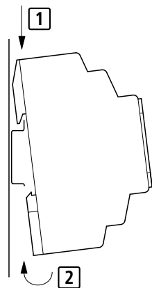
Abbildung 31:HutschieneMontage
