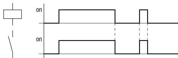
Abbildung 119:Wirkdiagramm „Schützfunktion“
