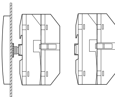
Abbildung 20: Netzteil-/CPU-Modul mit Ein-/Ausgangsmodule, links mit, rechts ohne Anzeige-/Bedieneinheit
